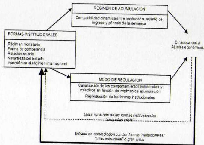
GRÁFICO 14. La arquitectura de las nociones de base de la teoría de la regulación
